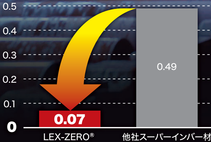
平均熱膨張係数の比較 (ppm/°C)
