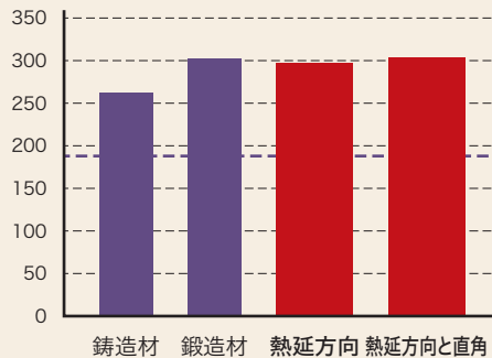
降伏点 (N/mm 2 )
