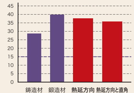
伸び (%)
