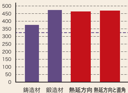
引張り強さ (MPa)
