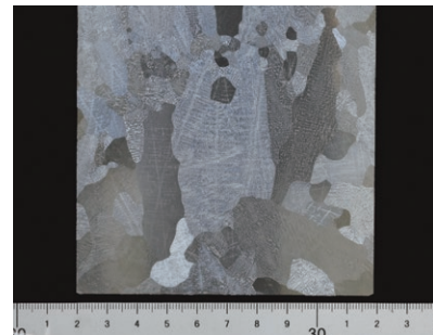
鋳造品_マクロ組織
