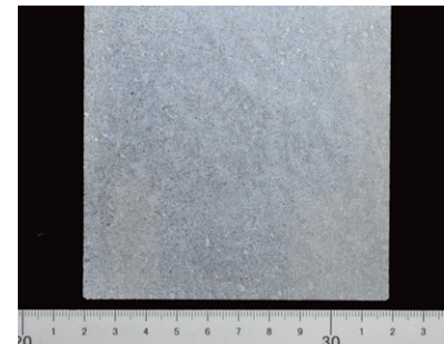
鍛造品_マクロ組織
